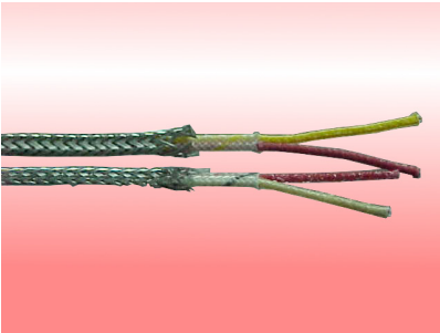
Serie: Fibra de Vidrio con Blindaje en Al304 (Ejemplo, N/P: F22-JX-FVBI)
