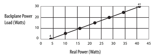
1756-PB30XT (DC)
