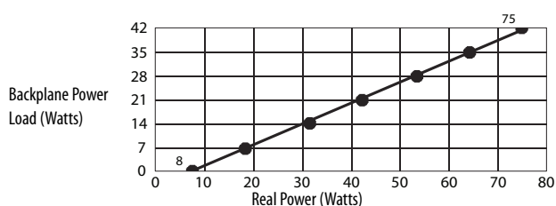
1756-PAXTR (AC)
