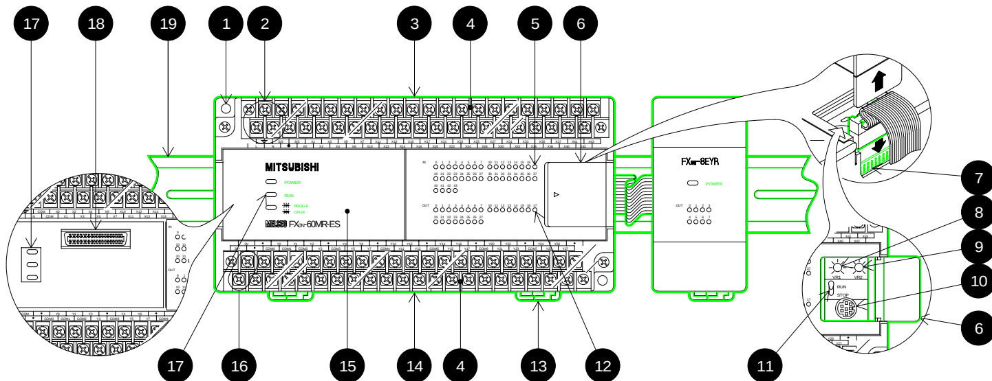
Figure: 3.1 ENG ⇨ Features of the FX0/FX0N PCs (FX0N shown) FRE ⇨ Caractéristiques des appareils FX0-/FX0N-API (à l'exemple du FX0N) GER ⇨ Merkmale der FX0-/FX0N-SPS (FX0N als Bildbeispiel) ITL ⇨ Caratteristiche dei PC FX0/FX0N (la figura rappresenta l'FX0N) ESP ⇨ Características de la unidad FX0-/FX0N-PC (FX0N como figura de ejemplo)
